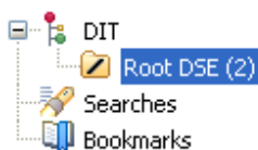
Slika 6 – OpenLdap struktura
